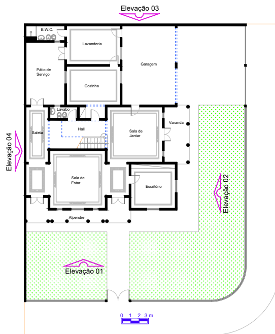
Térreo A = 226,82 m 2
