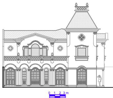
Elevação 01
