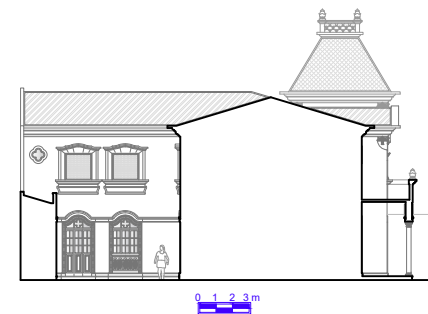
Elevação 04
